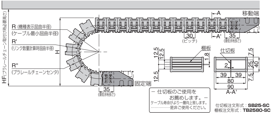
固定端取付寸法 (外周・内周取付共通)
