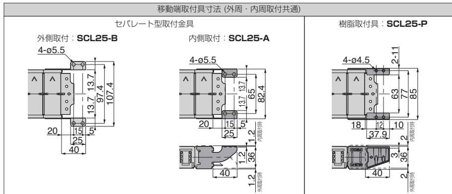
移動端取付寸法 (外周・内周取付共通)
