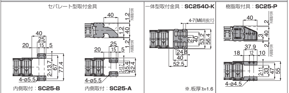
固定端取付寸法 (外周・内周取付共通)
