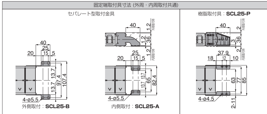
固定端取付寸法 (外周・内周取付共通)
