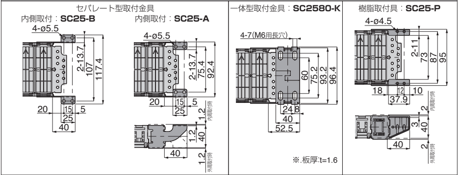
移動端取付寸法 (外周・内周取付共通)
