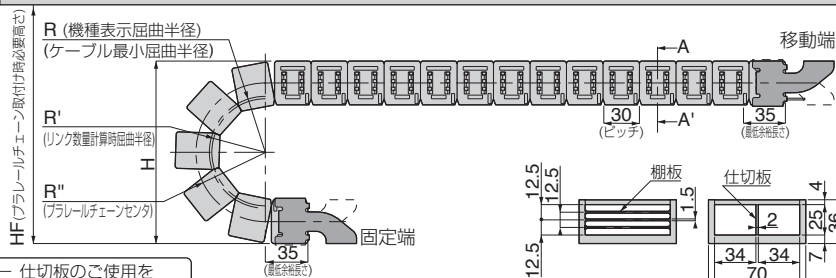
固定端取付寸法 (外周・内周取付共通)
