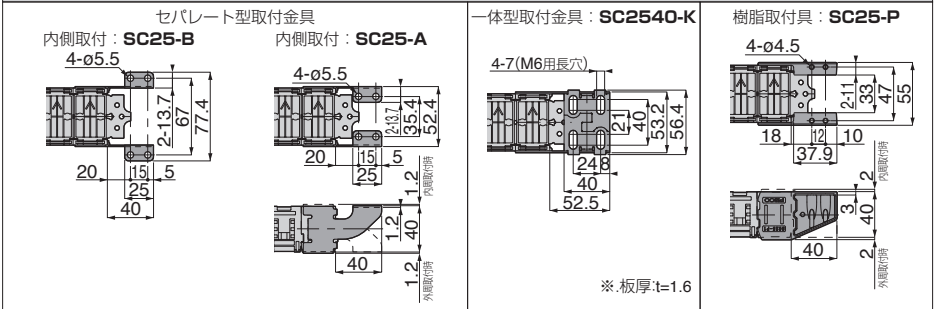
移動端取付寸法 (外周・内周取付共通)
