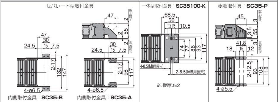
固定端取付具寸法 (外周・内周取付共通)
