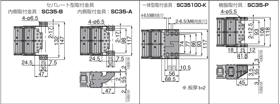
移動端取付具寸法 (外周・内周取付共通)
