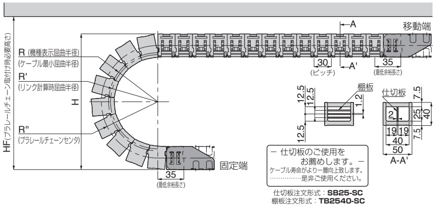
固定端取付寸法 (外周・内周取付共通)
