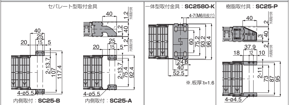
固定端取付寸法 (外周・内周取付共通)
